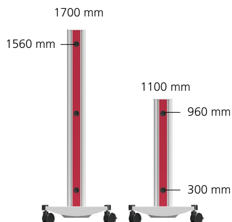
optionale Steckdosen
